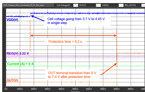
図 8-4. 過電圧保護
