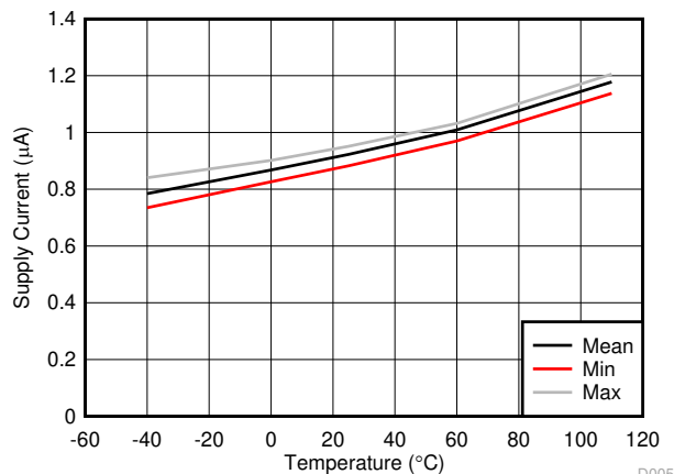
図 6-5. レギュレータがオフの I_{DD}
