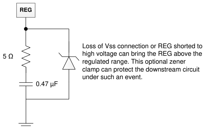
図 8-3. 5V ツェナー ダイオード
