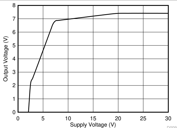
図 6-8. V_{OUT} と V_{DD} の関係
