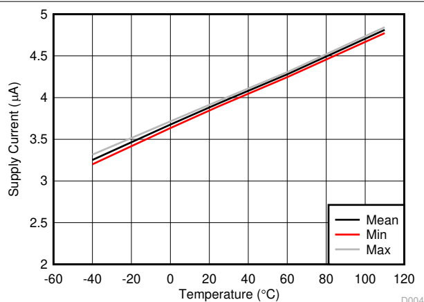
図 6-4. レギュレータがオンの I_{DD}
