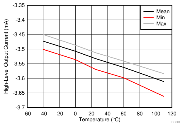
図 6-7. I_{OUTH} vs 温度
