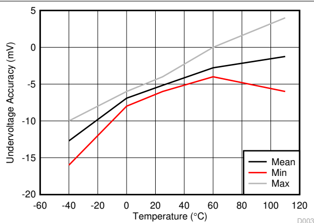
図 6-3. 低電圧の精度
