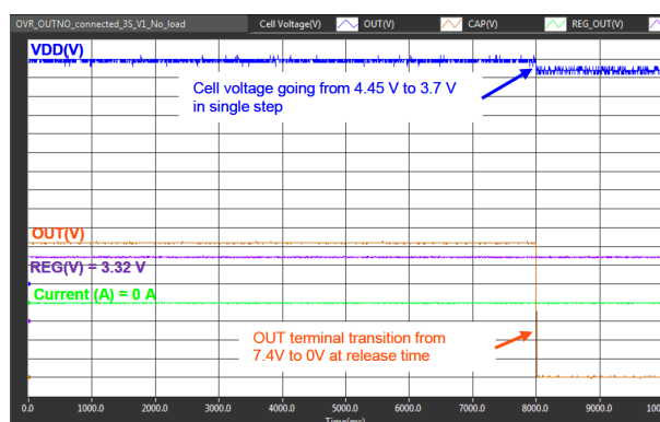
図 8-5. 過電圧保護リリース
