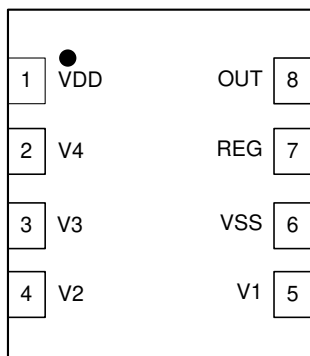
図 5-1. 2 ～ 4 直列の BQ2961 (上面図)
