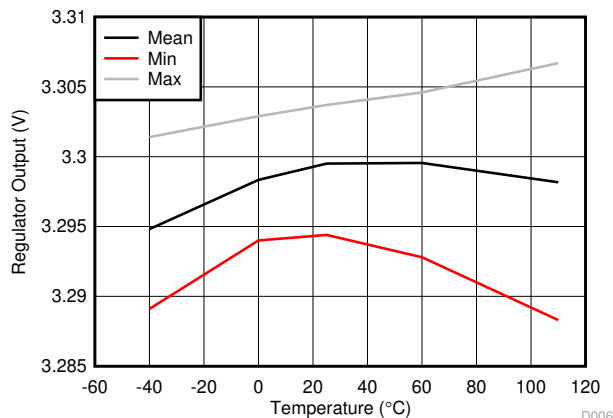
図 6-6. 負荷なしのレギュレータ出力
