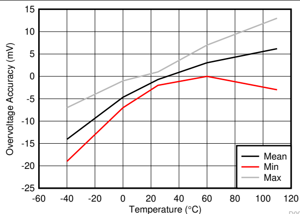
図 6-1. 過電圧スレッシュホールド ( V_{OV} ) と温度との関係
