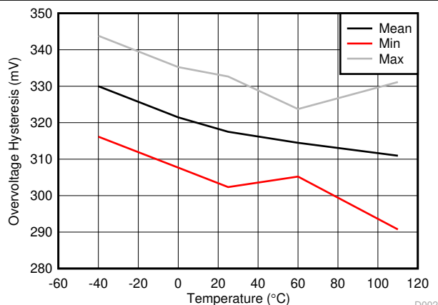
図 6-2. ヒステリシス V_{HYS} と温度との関係
